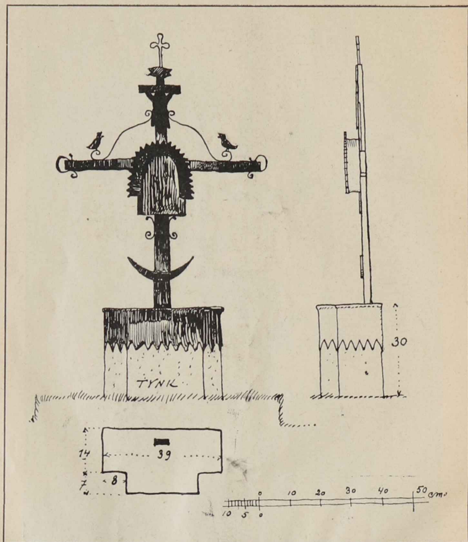
10. ŻELAZNY KRZYŻ NAGROBNY. POMYSŁ ROMUALDA GUTTA.
